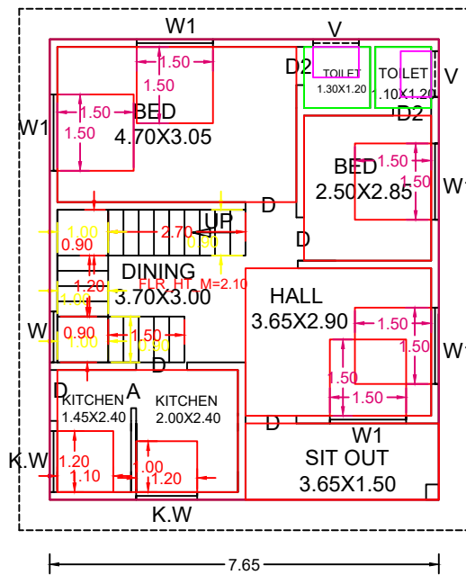
G.F.PLAN
