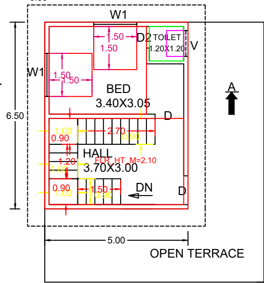
F.F.PLAN
