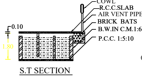
S.T. SECTION
