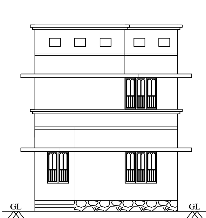
ELEVATION
