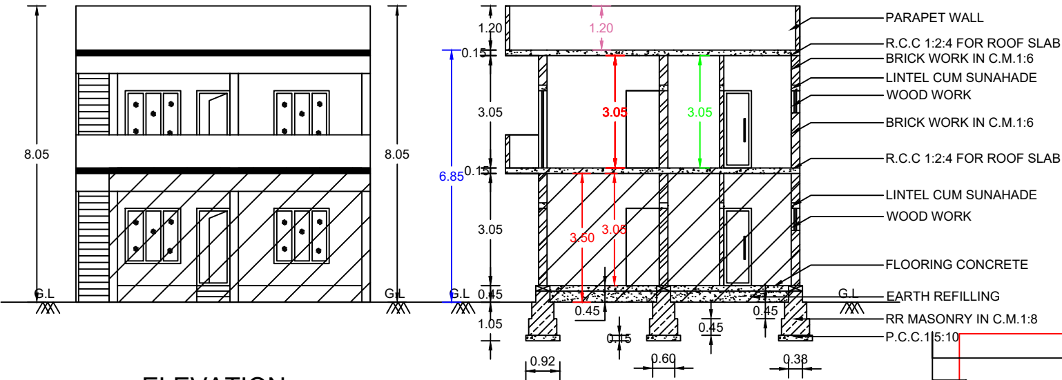
ELEVATION
