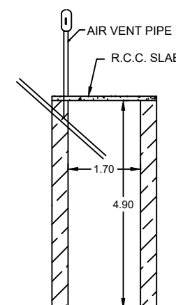
SOAK PIT
