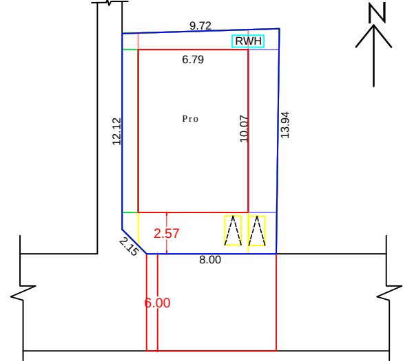
SCALE 1:100 SITE PLAN
