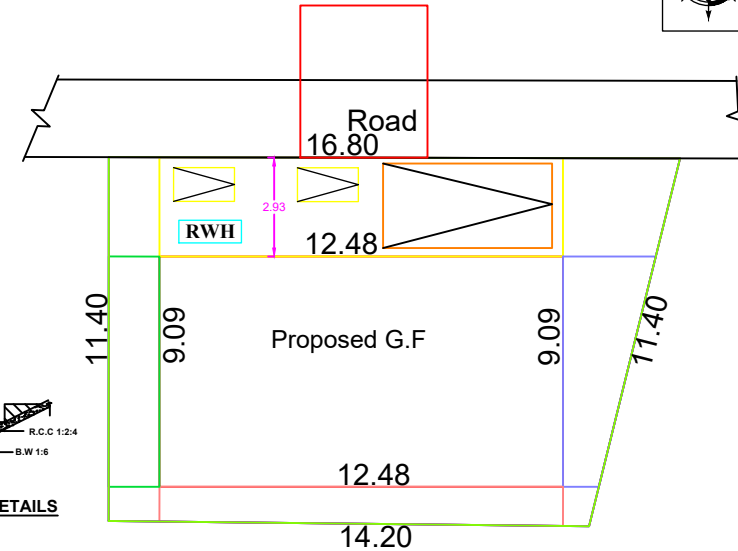
SITE PLAN 1:100
