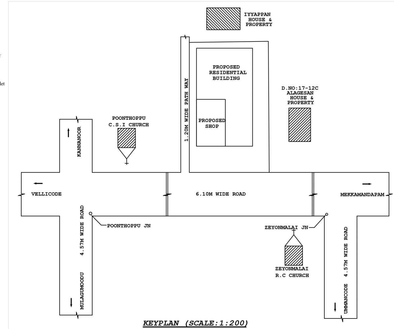
KEYPLAN (SCALE:1:200)
