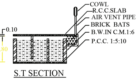
S.T SECTION
