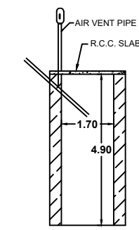
SOAK PIT
