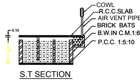
S.T. SECTION
