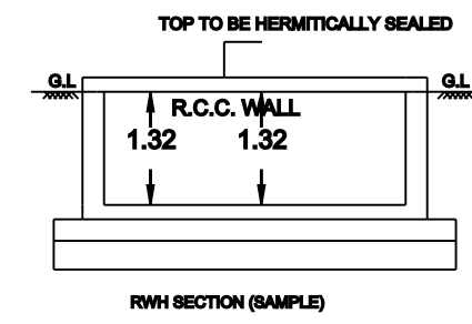
RCC WALL (1.00)
