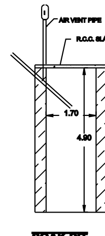
SOAK PIT
