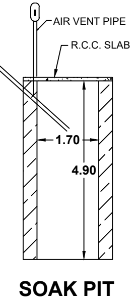
SOAK PIT
