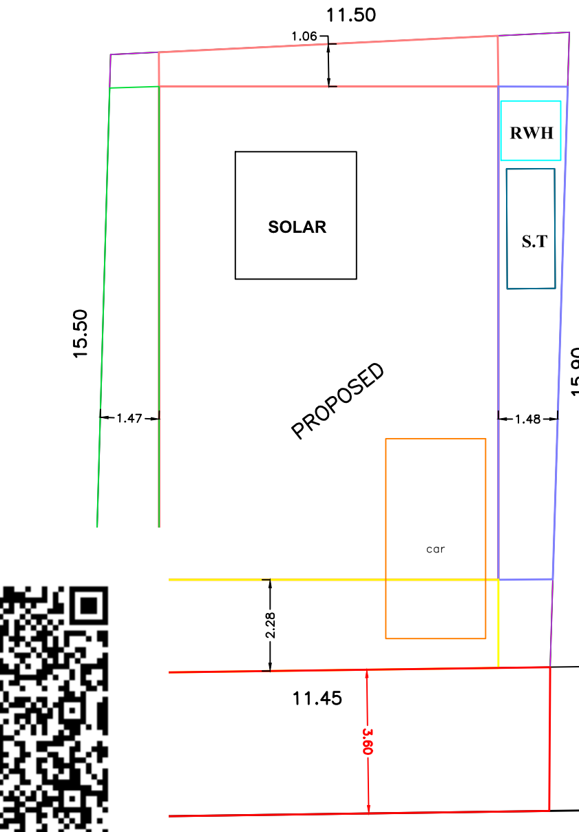
SITE PLAN ;1:100
