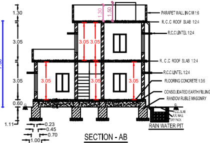
SECTION - AB
