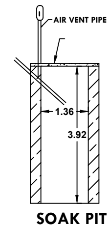
SOAK PIT
