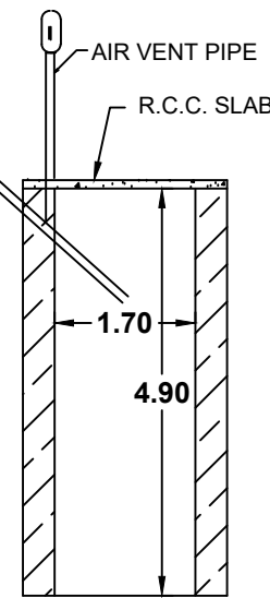
SOAK PIT
