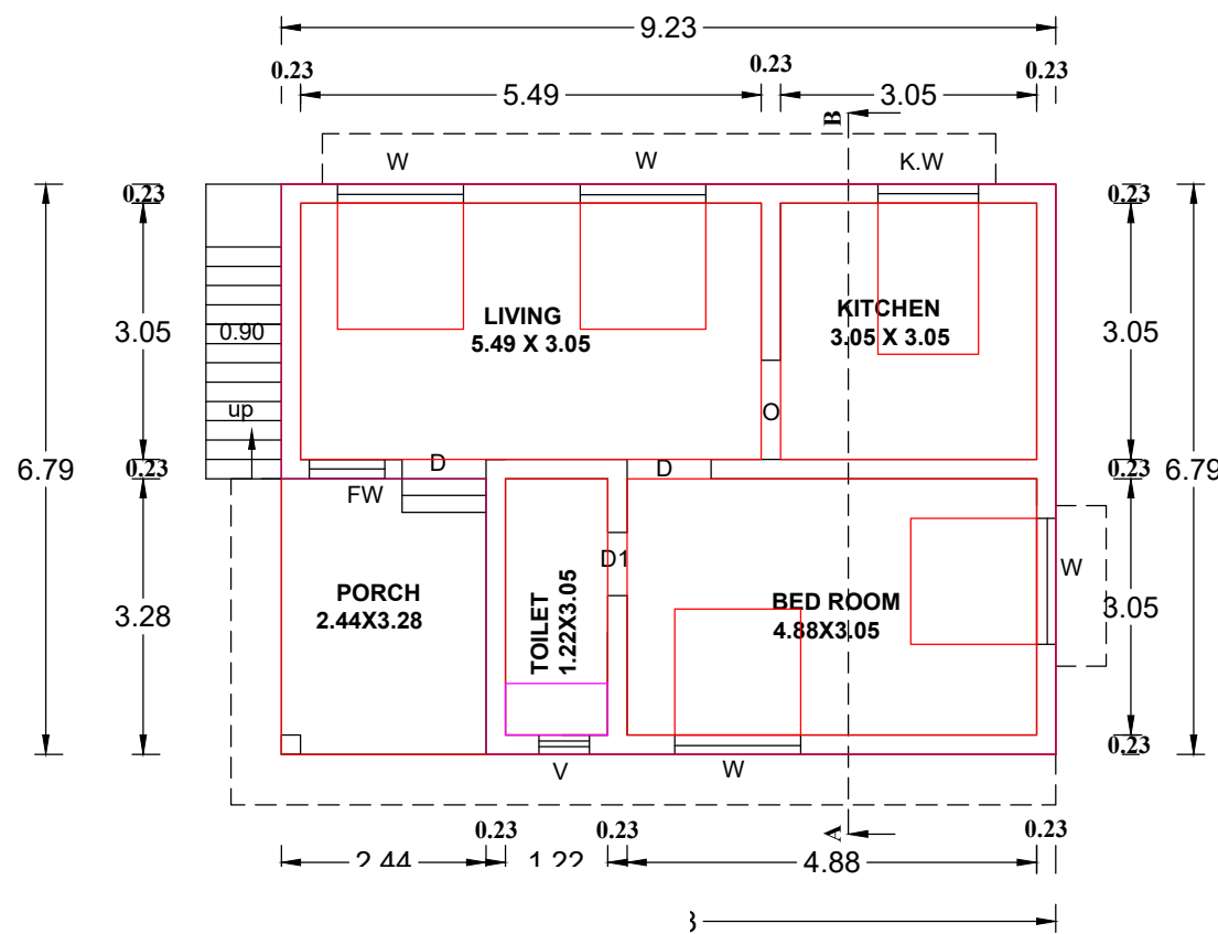
DOOR PLAN
