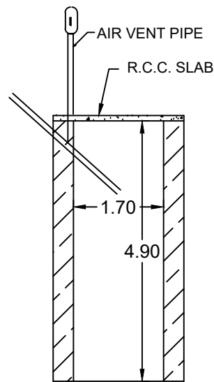
SOAK PIT
