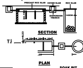
SOAK PIT
