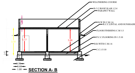
SECTION A-B
