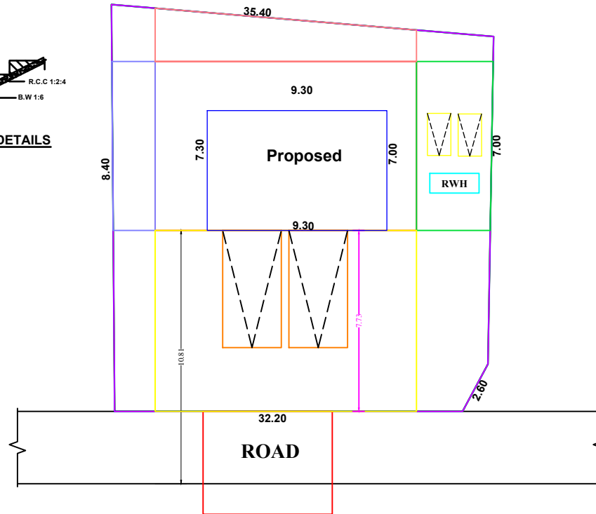
SITE PLAN 1:100
