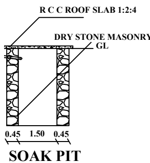
SOAK PIT
