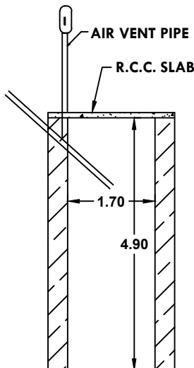
SOAK PIT
