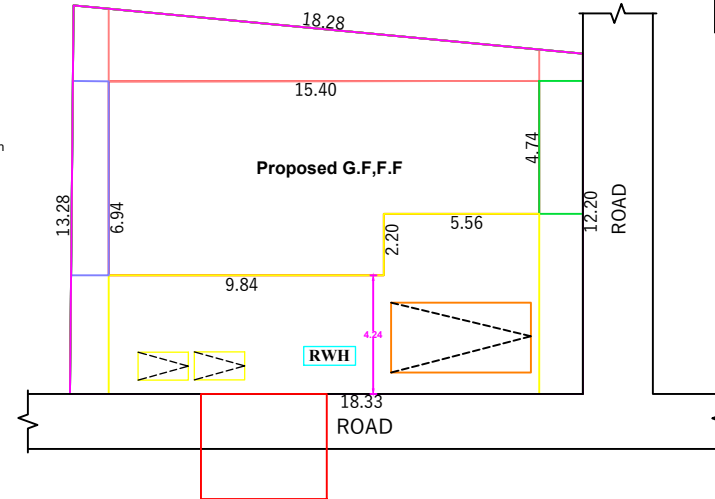
SITE PLAN 1:100
