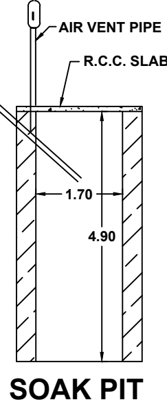
SOAK PIT
