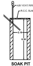
SOAK PIT
