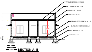
SECTION A-B
