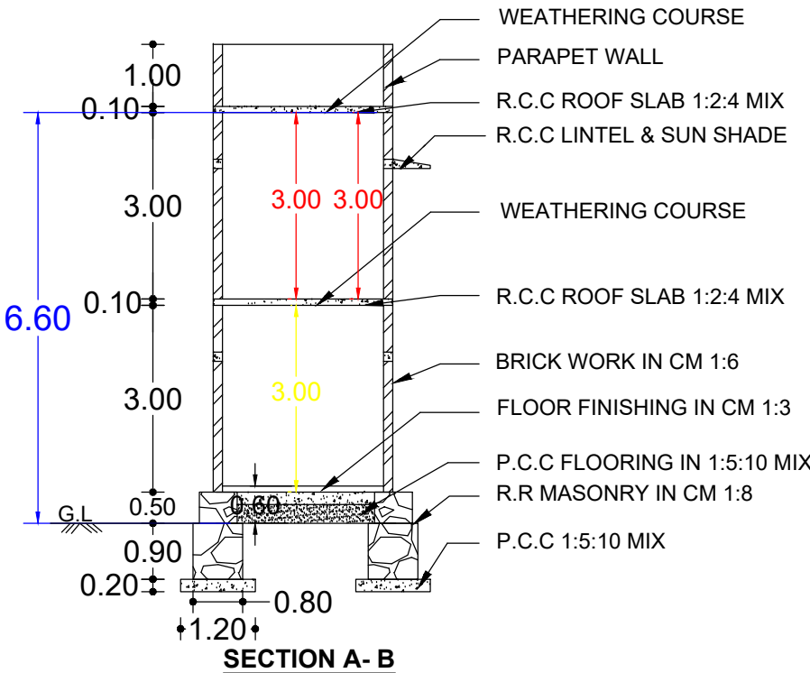
SECTION A-B
