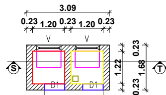
TOILET PLAN
