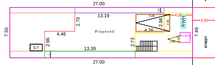
SITE PLAN SCALE 1:100
