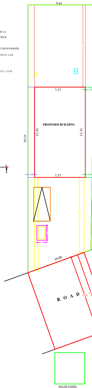
SITE PLAN SCALE 1:100
