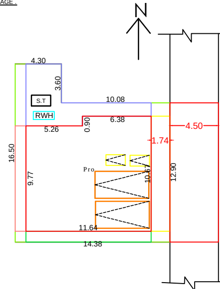
SCALE 1:100 SITE PLAN
