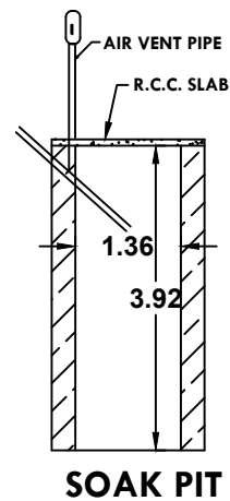
SOAK PIT
