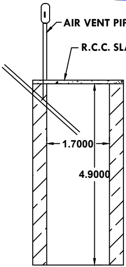
SOAK PIT
