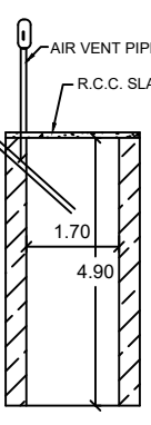
SOAKPIT
