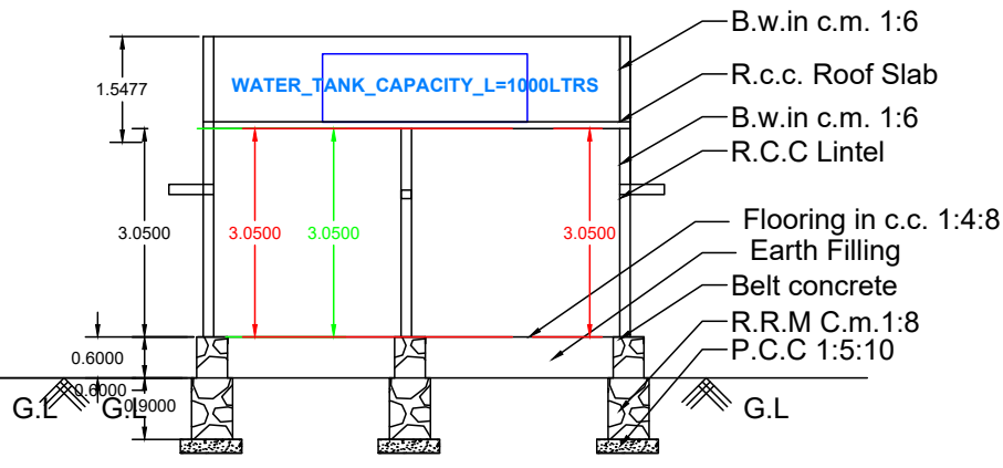
SECTION A-B
