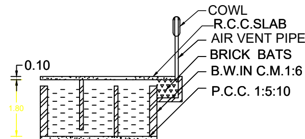
S.T. SECTION
