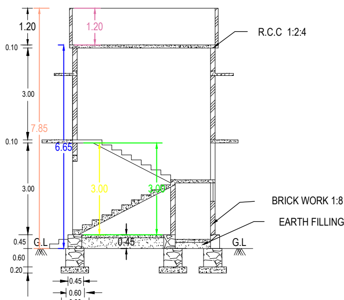
SECTION A-B
