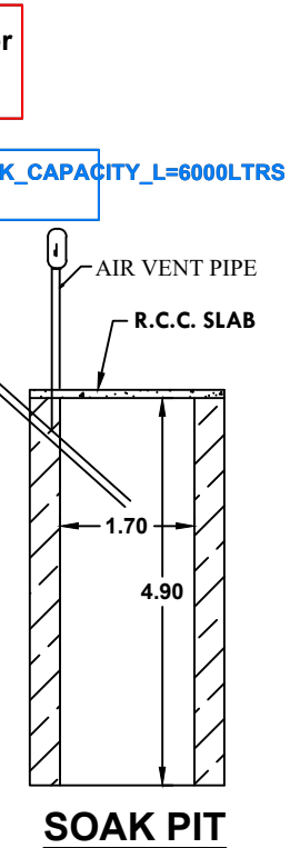
SOAK PIT
