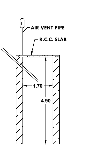
SOAK PIT
