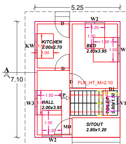
G.F.PLAN (R.C.C.ROOF
