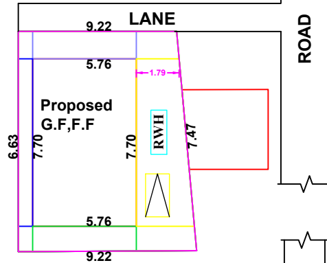
SITE PLAN 1:100
