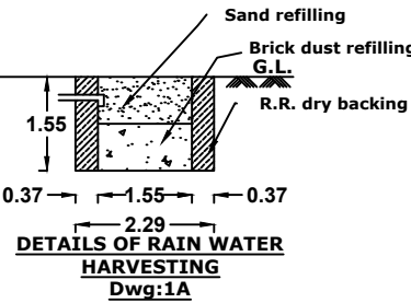
SOAK PIT
