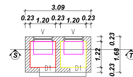
TOILET PLAN
