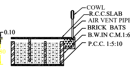
S.T SECTION
