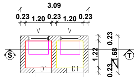
TOILET PLAN
