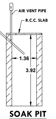
SOAK PIT
