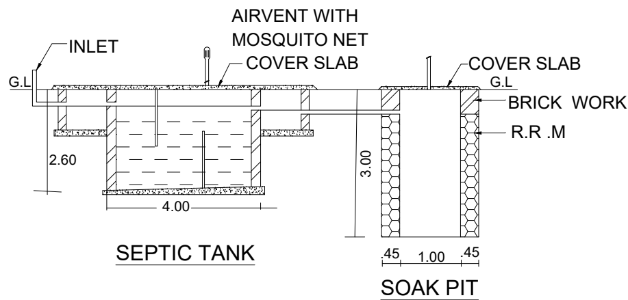
SOAK PIT
