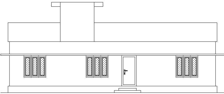
ELEVATION
