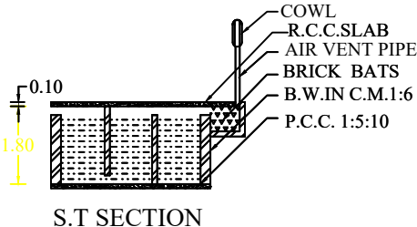
S.T SECTION
