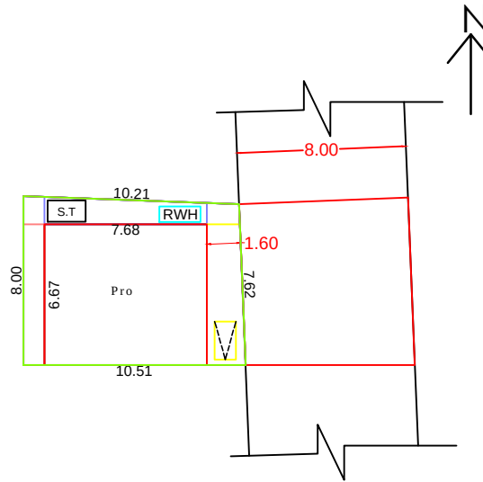
SCALE 1:100 SITE PLAN
