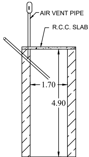
SOAK PIT
