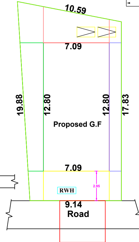
SITE PLAN 1:100
